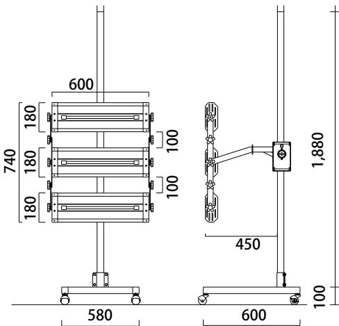
【寸法図】
